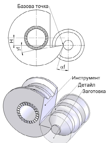
Фиг. 1. Кръгл профилен нож
