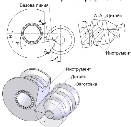
Фиг. 2. Кръгл профилен нож с базова линия
