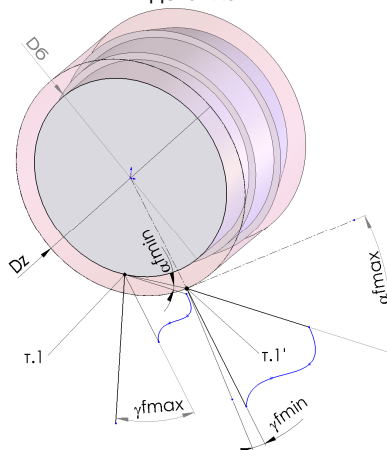
Фиг. 4. Профилен нож с тангенциално подаване
