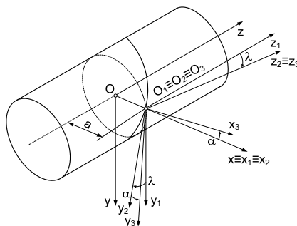
Фиг. 5. Координатни системи при профилиране на резбонарезни ножове
